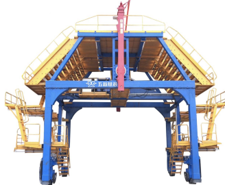
防水板/钢筋作业台车
