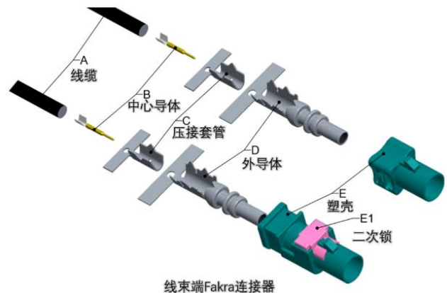
图表45：线束端 Fakra 连接器结构
