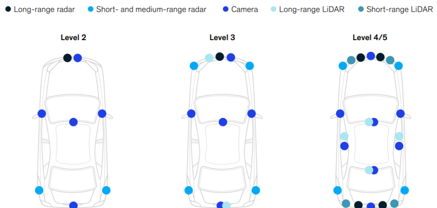
图表21: 高级别智能驾驶要配置更多传感器
