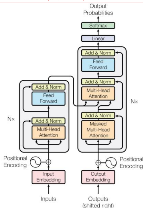
图表 67: Transformer 架构示意图
