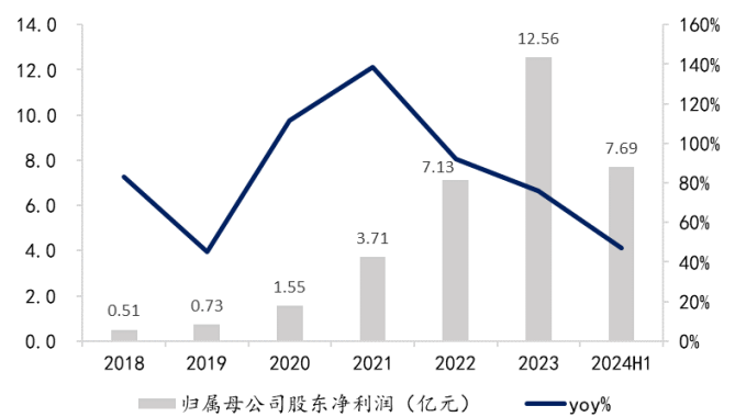
图2：2024H1 归母净利润为 7.69 亿元，同比+47.2%
