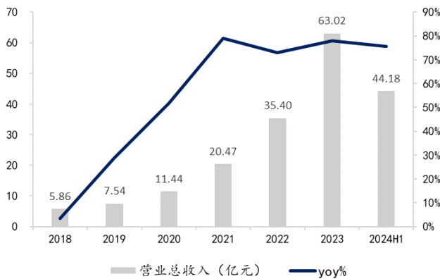
图1：公司 2024H1 实现营收 44.18 亿元，同比+75.5%
