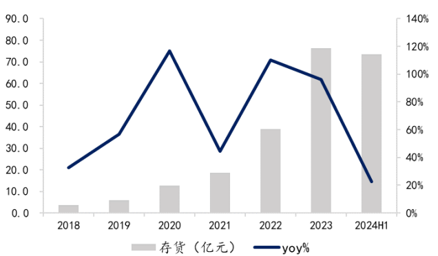
图6: 2024H1 存货为 73.4 亿元，环比-4%
