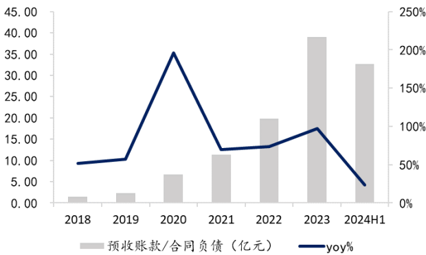
图5: 2024H1 合同负债为 32.6 亿元，环比-17%
