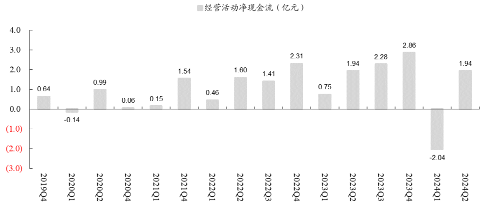
图7：2024Q2 经营性现金流回正至 1.94 亿元
